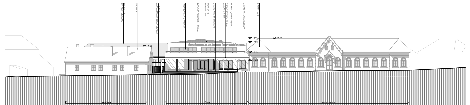
Iskola utcai homlokzat
